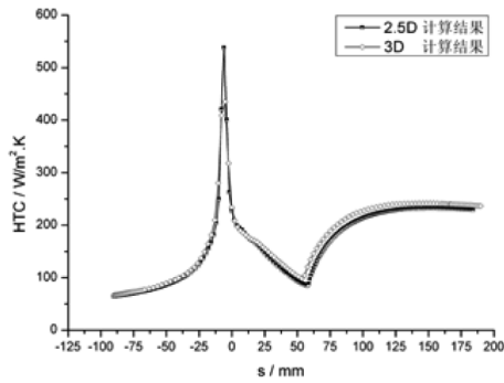
图5 2.5D及3D模型中间截面对流换热系数
