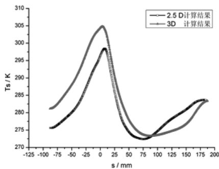
图6 2.5D及3D模型中间截面表面温度分布
